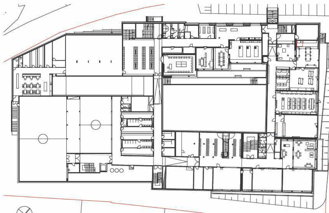
Grundriss Erdgeschoß
