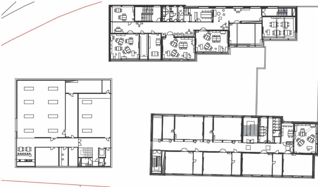
Grundriss 1. Obergeschoß
